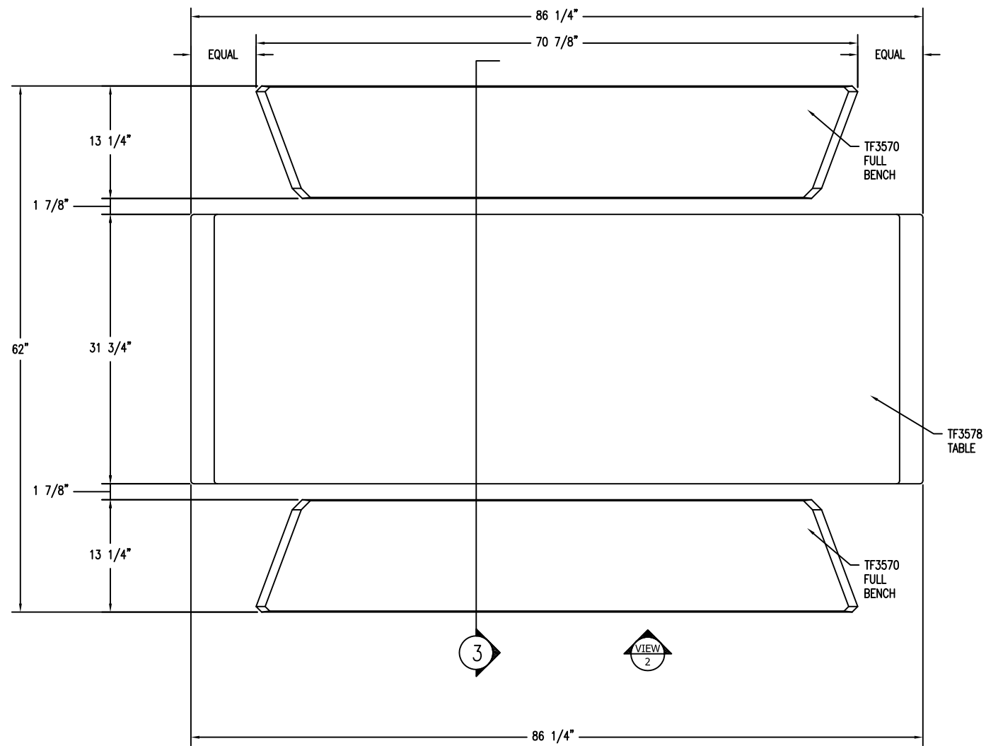
1 TOP VIEW Scale: 1/8" = 1"
