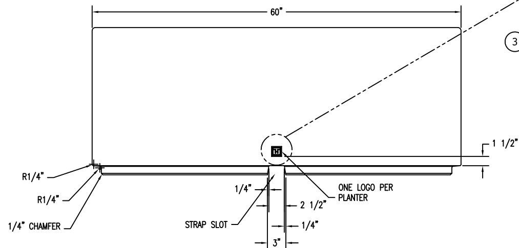
2 ELEVATION Scale: 1/8" = 1"
