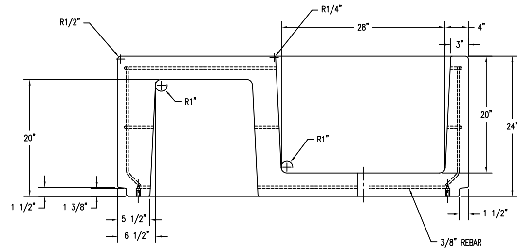
5 CROSS SECTION Scale: 1/8" = 1"
