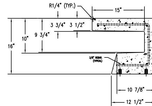
5 SECTION Scale: 1/4" = 1"
