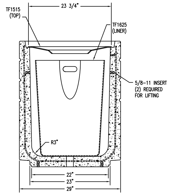
3 SECTION Scale: 1 1/2" = 1'-0"
