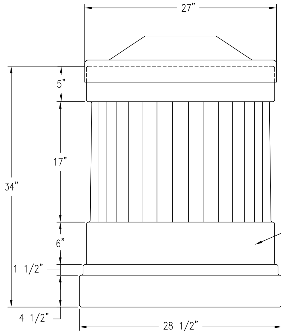
1 ELEVATION VIEW Scale: 1/8" = 1"
