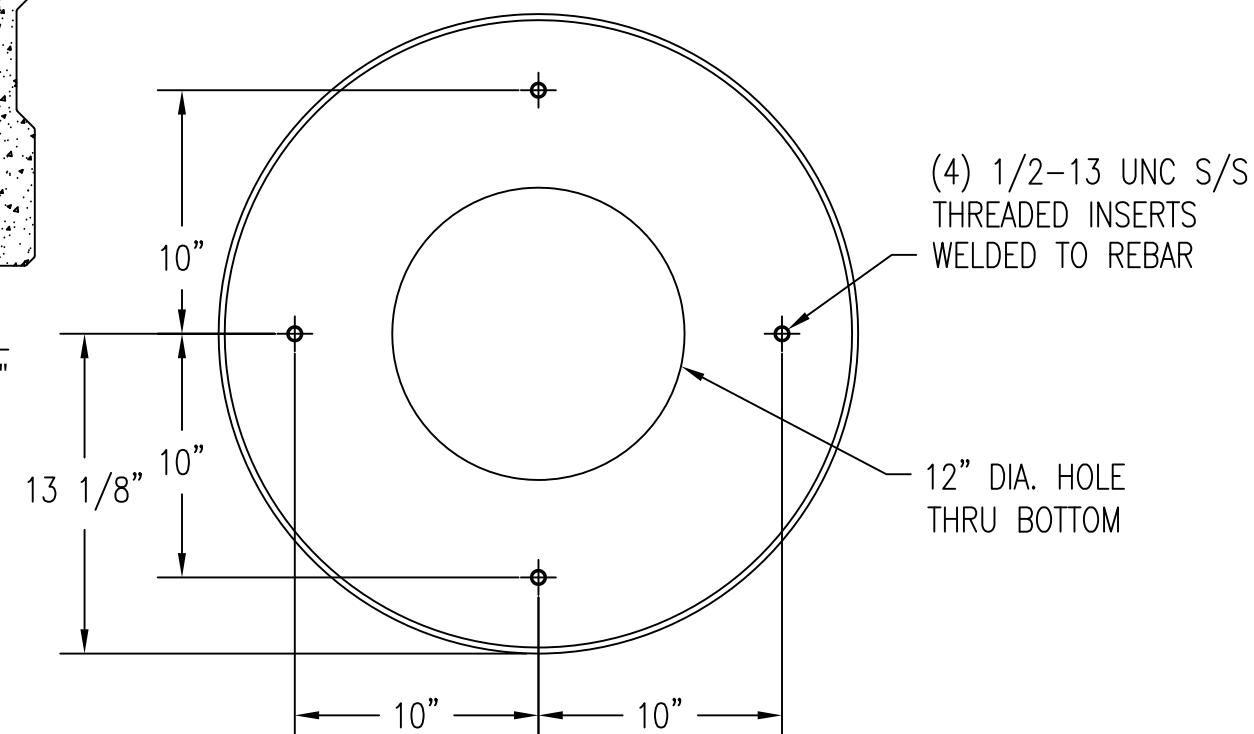
4 BOTTOM VIEW Scale: 1/8" = 1"
