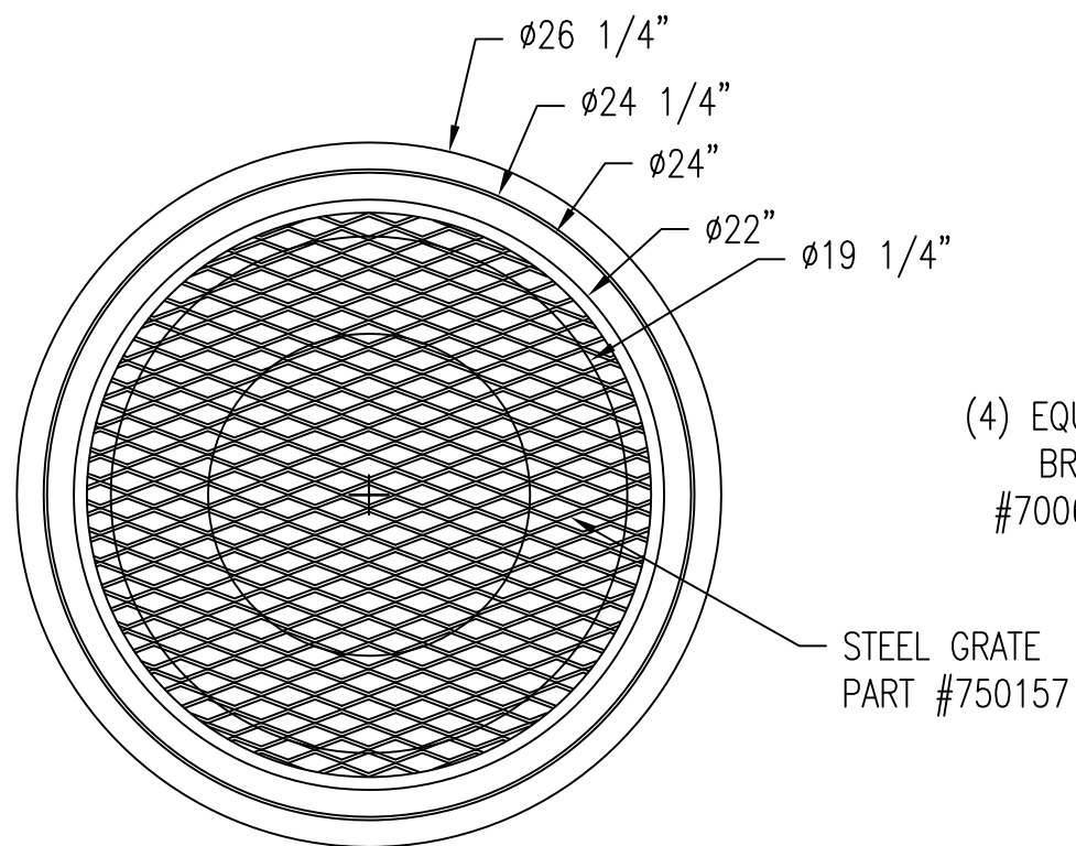
1 TOP VIEW Scale: 1/8" = 1"
