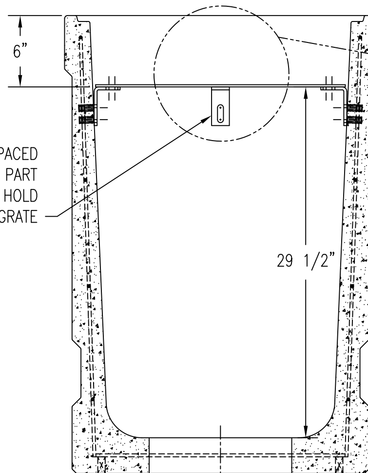
3 CROSS SECTION Scale: 1/8" = 1"
