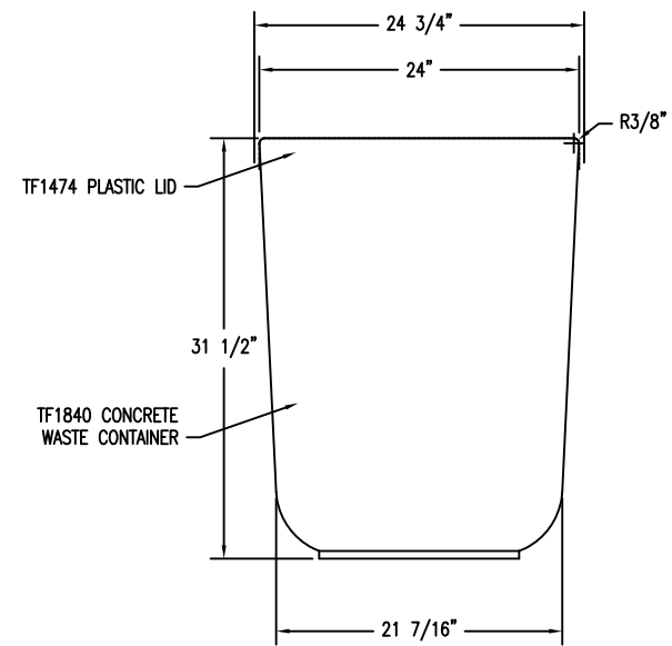
2 ELEVATION VIEW Scale: 1/8" = 1"
