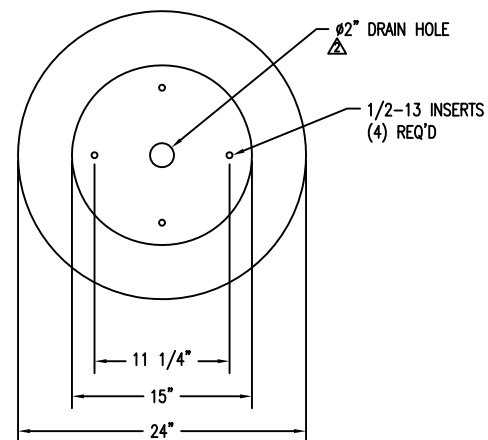
3 BOTTOM VIEW Scale: 1/8" = 1"
