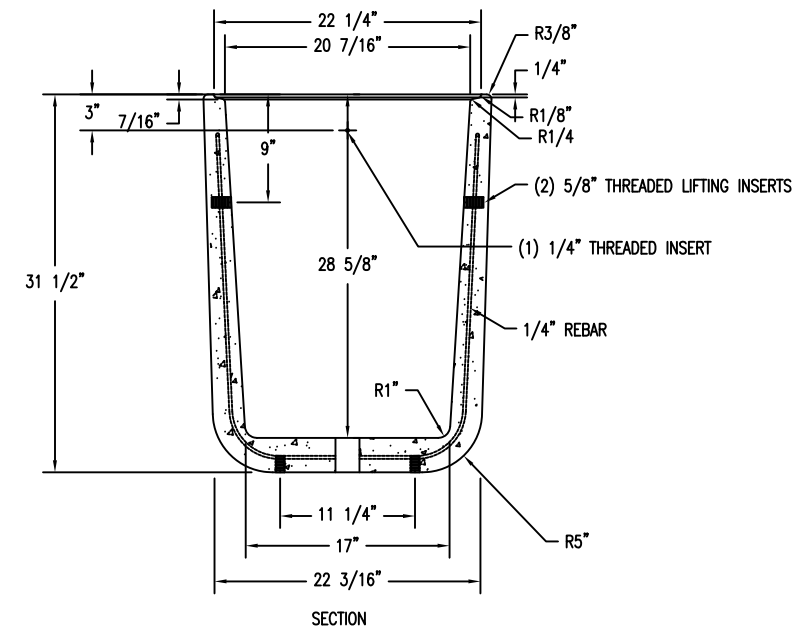
4 SECTION VIEW Scale: 1/8" = 1"
