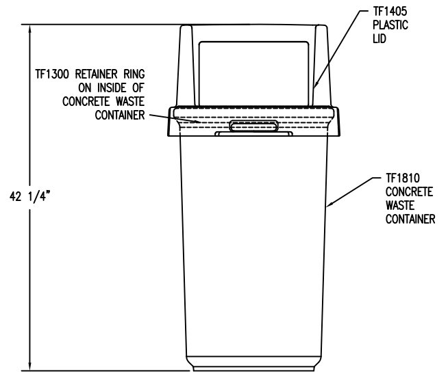
2 ELEVATION VIEW Scale: 1/8" = 1"
