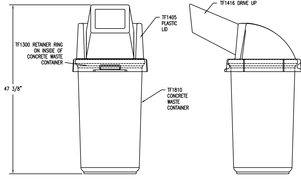
2 ELEVATION VIEW Scale: 1/8" = 1"
