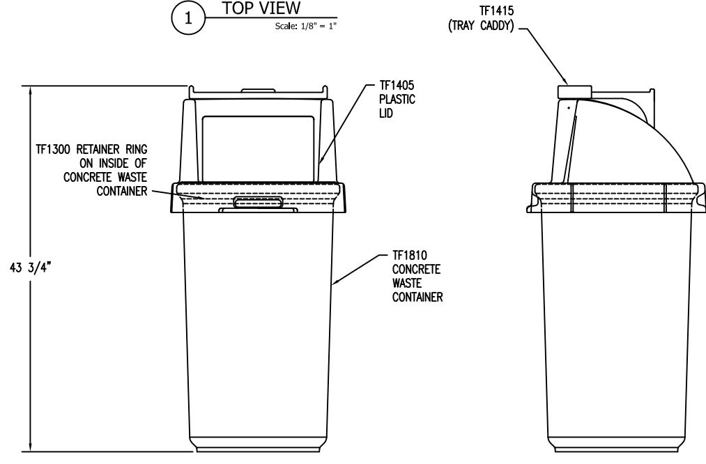
2 ELEVATION VIEW Scale: 1/8" = 1"
