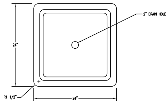
1 TOP VIEW Scale: 1/8" = 1"
