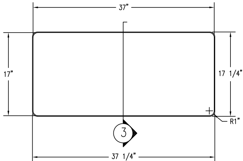
1 TOP VIEW Scale: 1/8" = 1"
