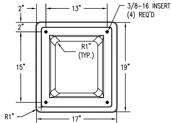
4 BOTTOM VIEW Scale: 1/8" = 1"
