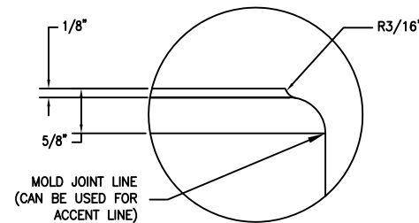
5 DETAIL Scale: 1/8" = 1"
