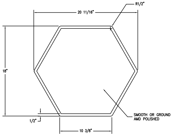
1 TOP VIEW Scale: 1/8" = 1"
