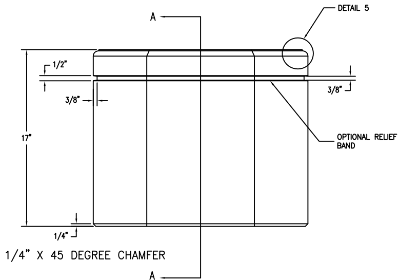
2 ELEVATION VIEW Scale: 1/8" = 1"
