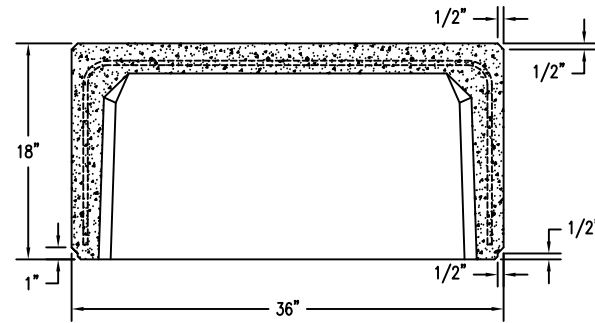
3 SECTION VIEW Scale: 1/8" = 1"
