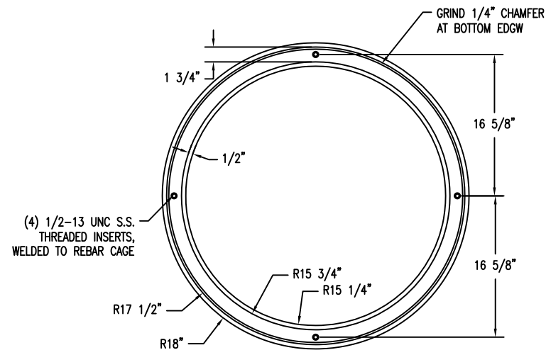
4 BOTTOM VIEW Scale: 1/8" = 1"
