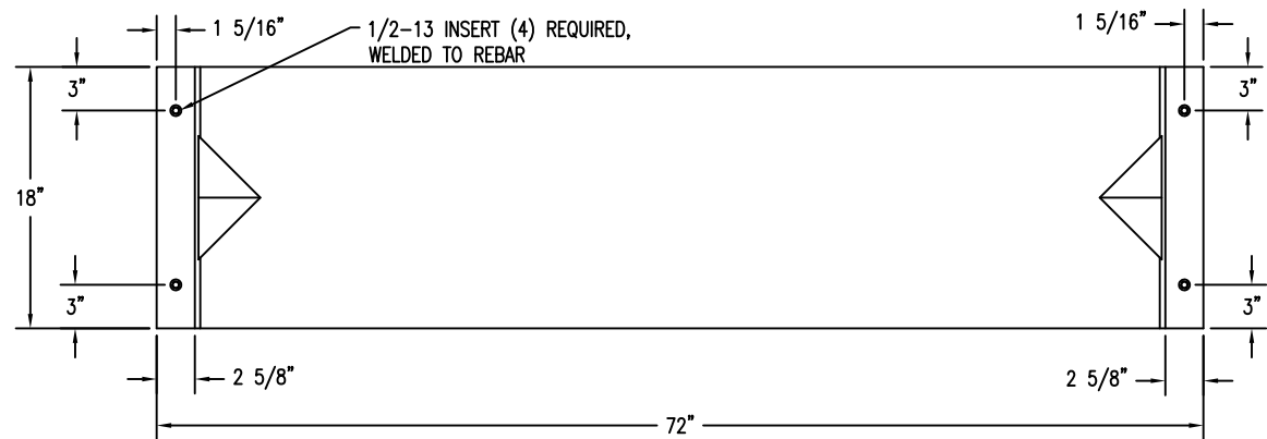
3 BOTTOM VIEW Scale: 1/8" = 1"
