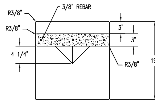
4 SECTION VIEW Scale: 1/8" = 1"
