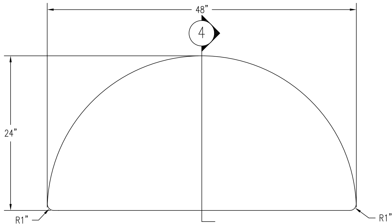
1 TOP VIEW Scale: 1/8" = 1"
