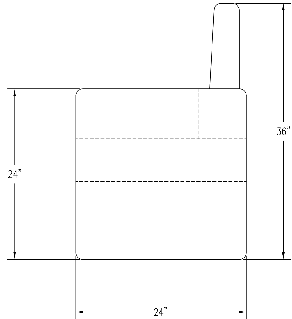
2 SIDE ELEVATION Scale: 1/8" = "1"
