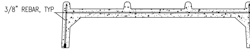
4 SECTION VI Scale: 1/16" = 1"
