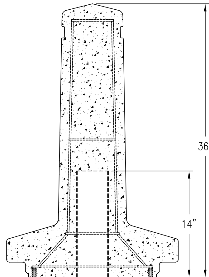
3 SECTION VIEW Scale: 1/8" = 1"
