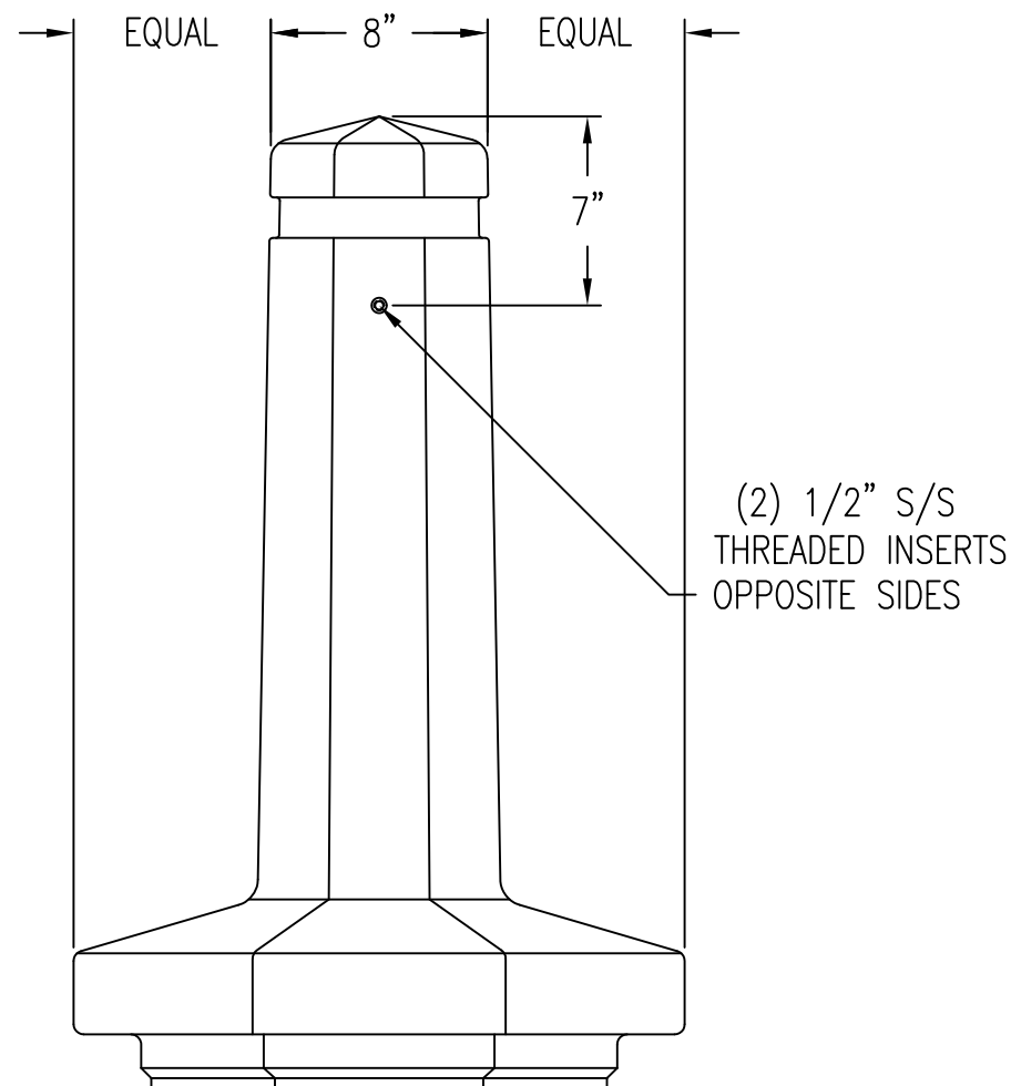
2 ELEVATION VIEW Scale: 1/8" = 1"
