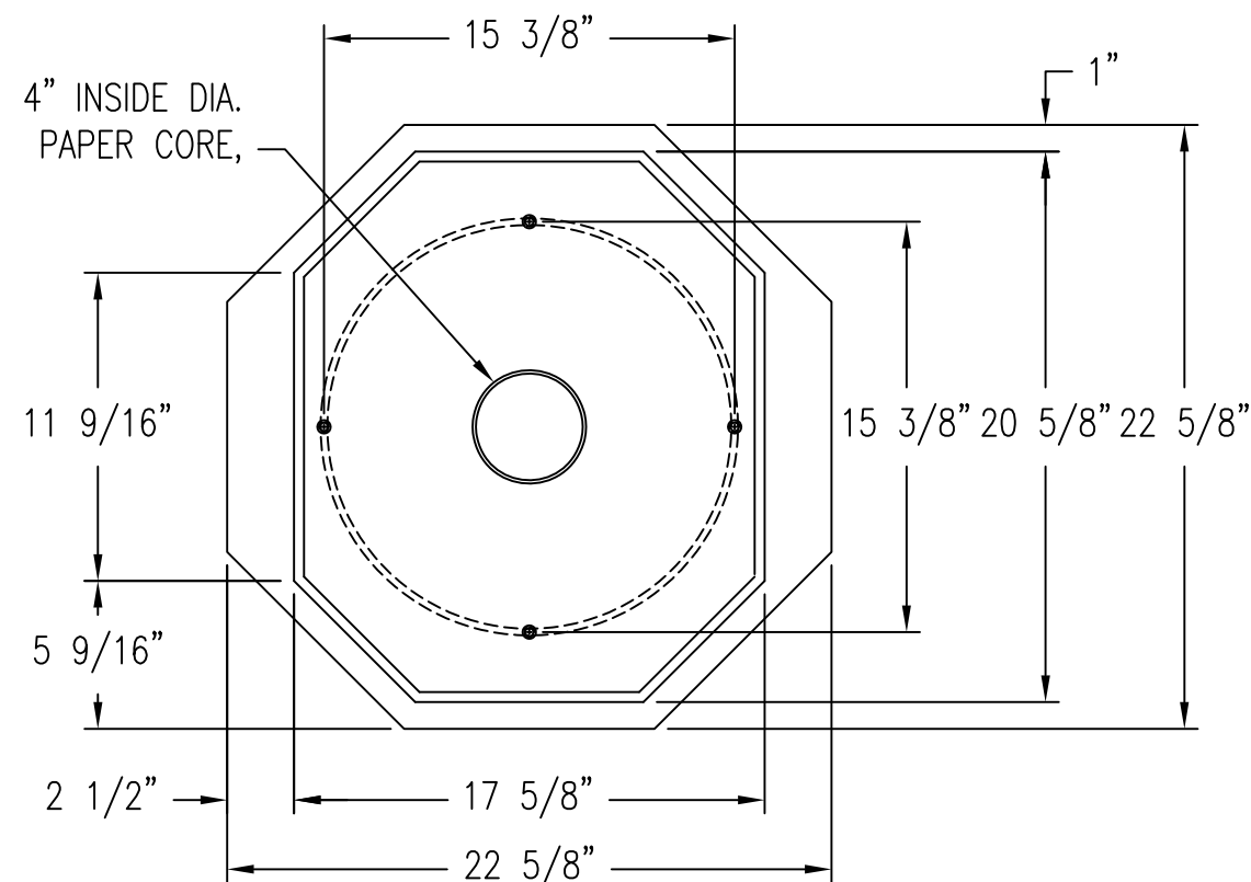
4 BOTTOM VIEW Scale: 1/8" = 1"
